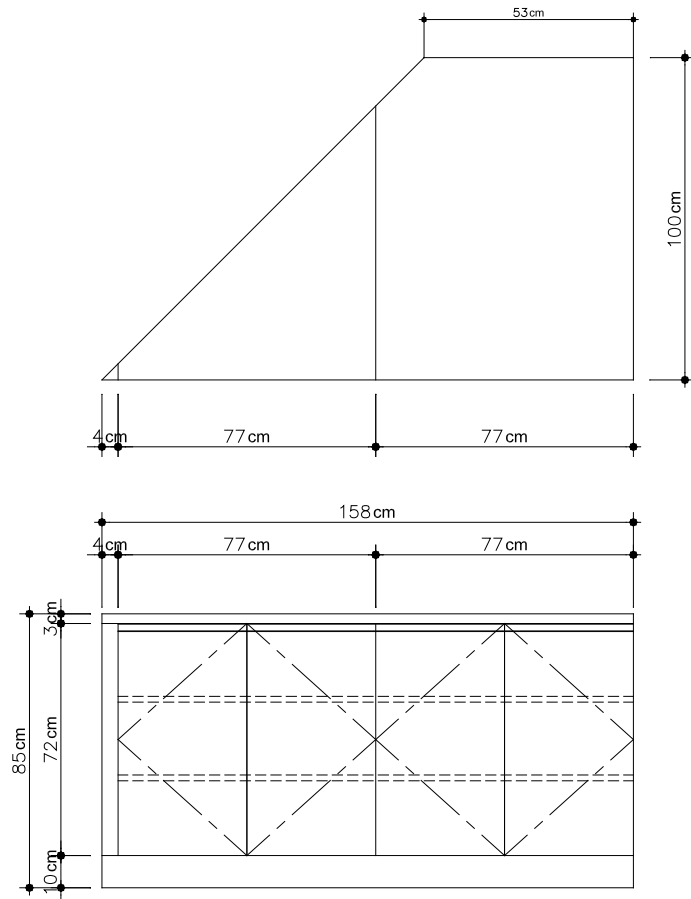
圖14 置物櫃A型(新店市公所站)
