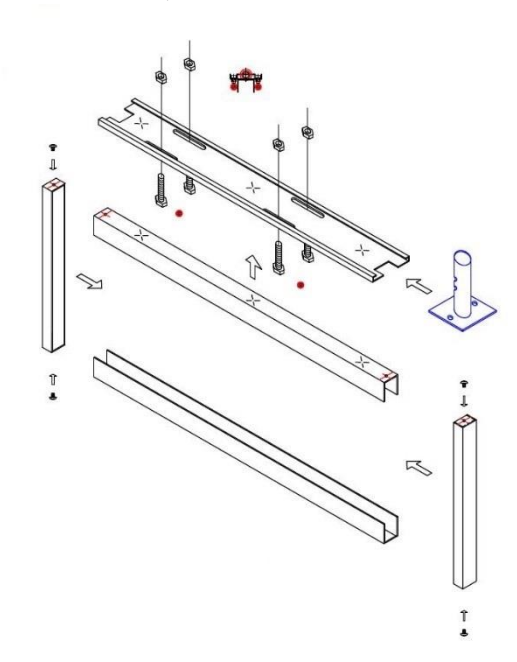
圖一：不銹鋼燈框設計圖
