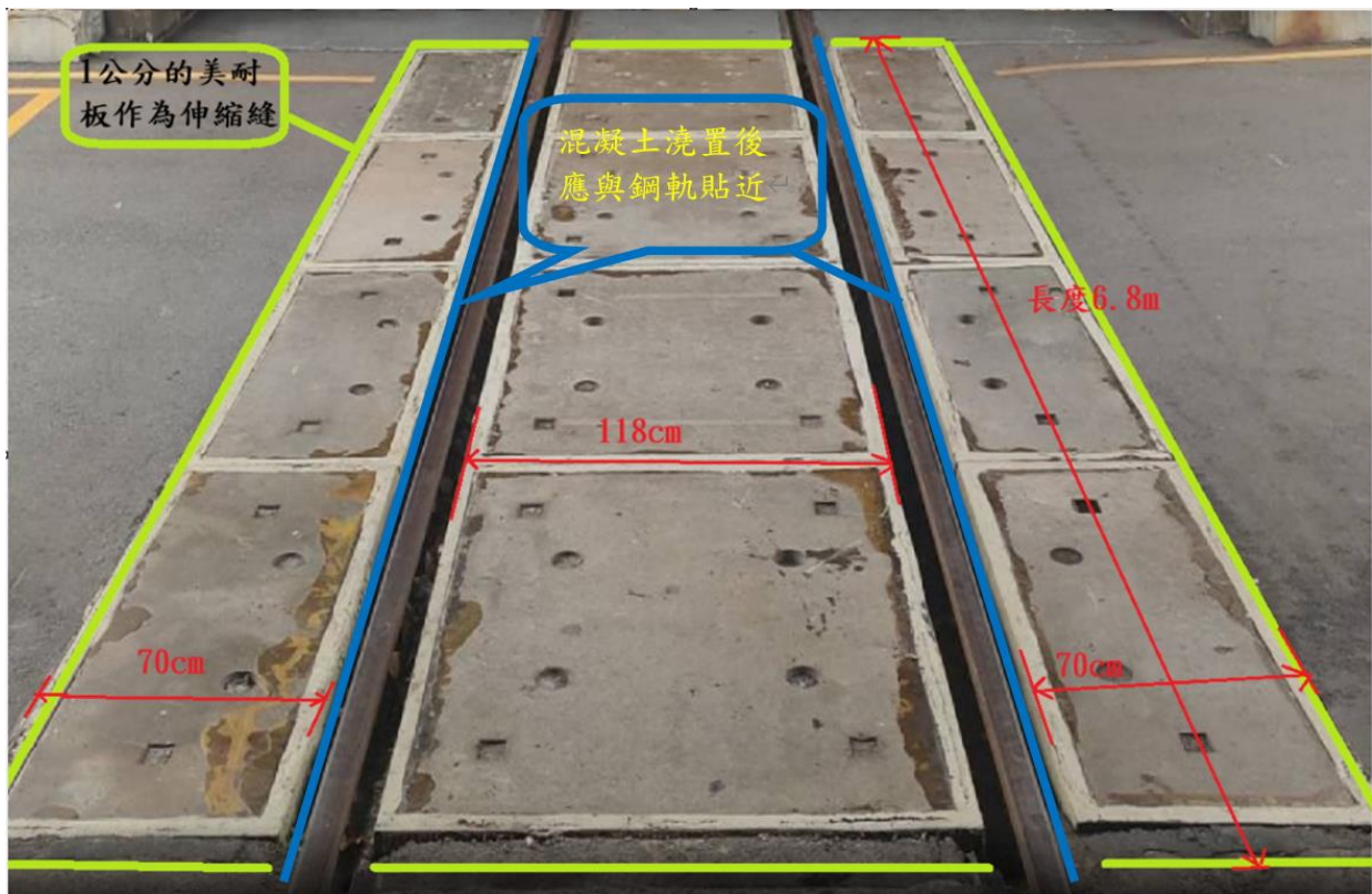
圖 2-澆置高度 15 公分(含)以上，混凝土澆置完成後不得干涉車輛行駛
