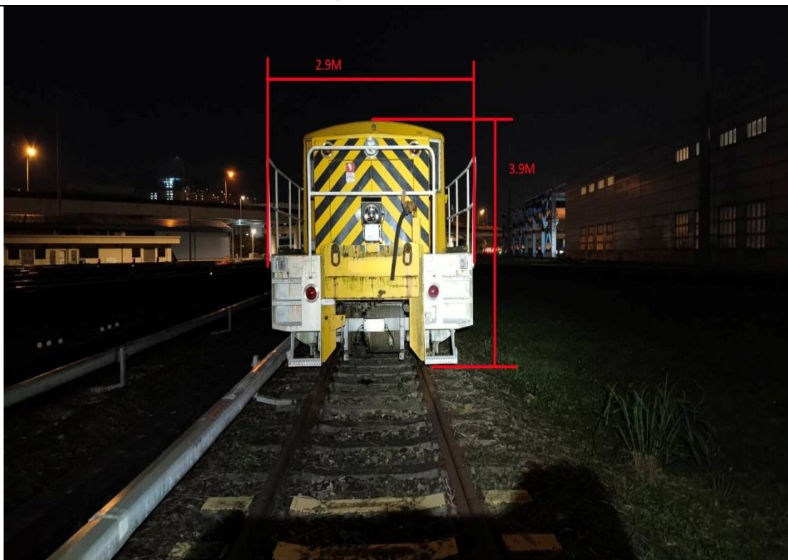
機車頭正面尺寸
