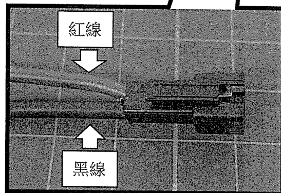
圖 3-2：2P 快拆公接頭
