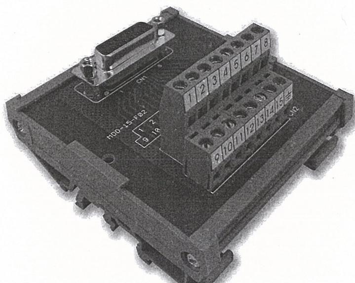
參考圖示：D-Sub 聯結器
