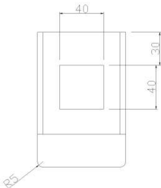
圖 5、無線電放置盒前視圖
