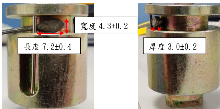
圖二、焊點尺寸示意圖(單位：mm)
